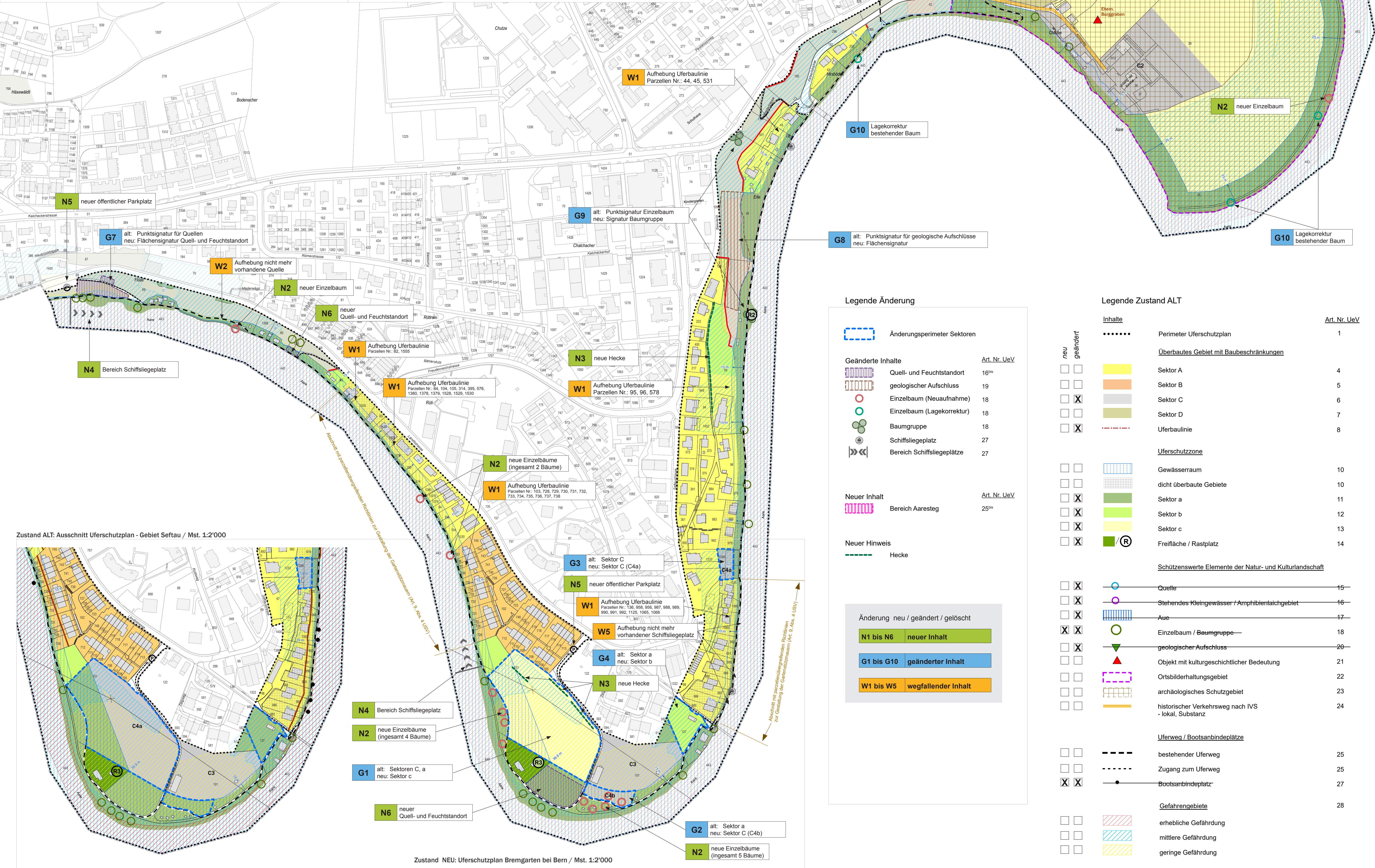
Zustand NEU: Uferschutzplan Bremgarten bei Bern / Mst. 1:2'000
